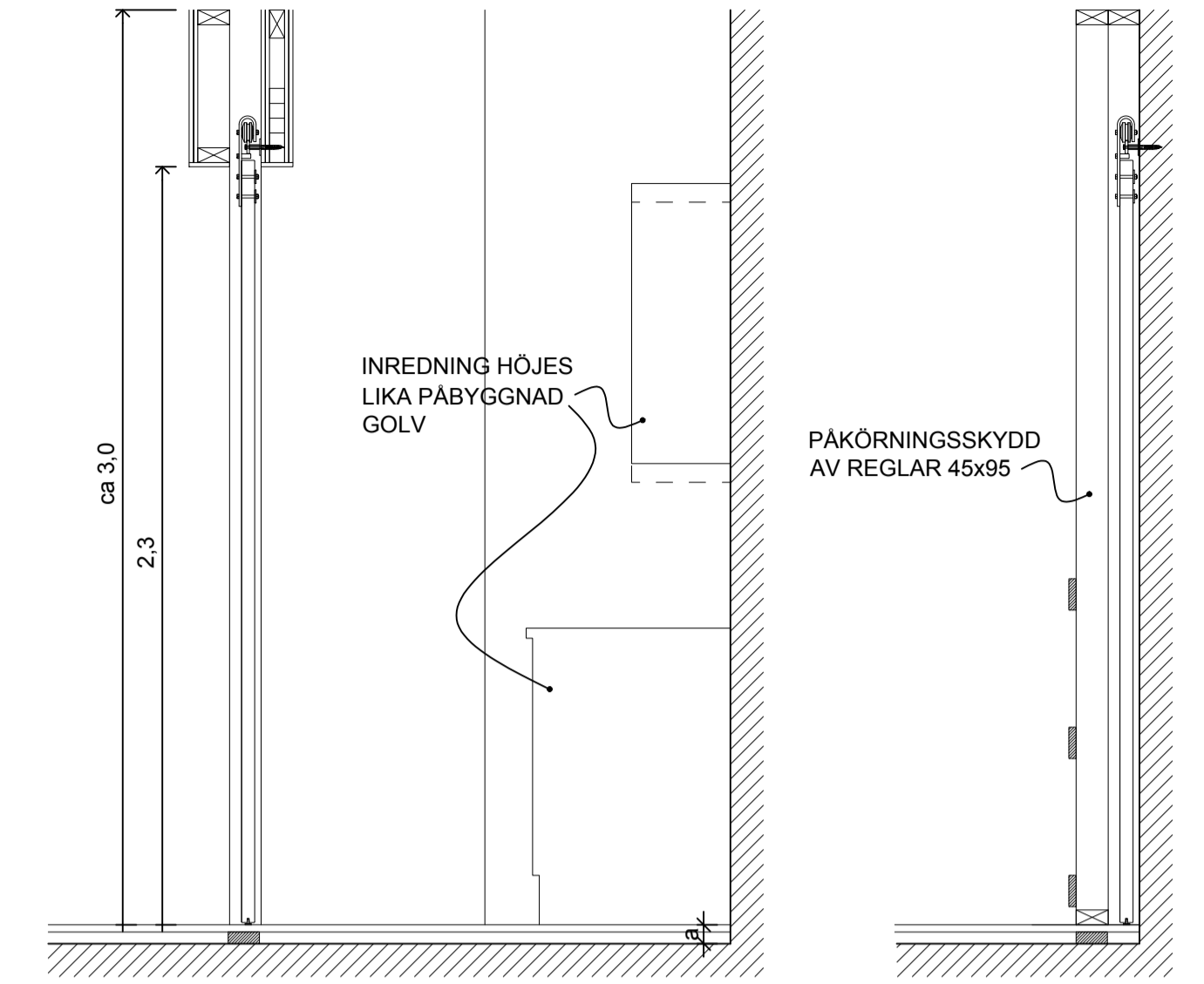
SEKTION A-A Skala 1:20
